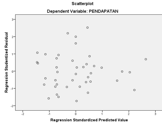
Gambar 2 Uji Heterokedastisitas
